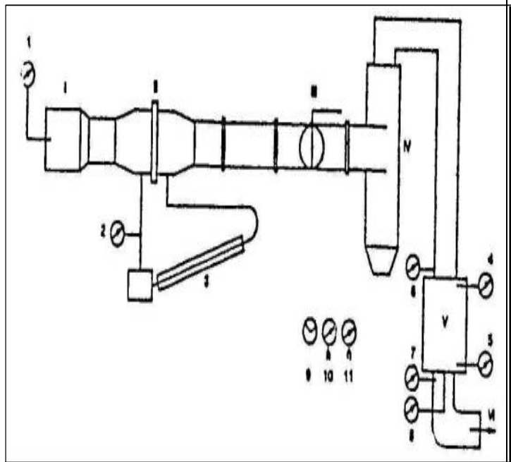
圖十 CVS 系統確認設備配置圖
