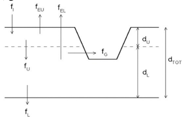
圖 2 地下水二層模式示意圖
