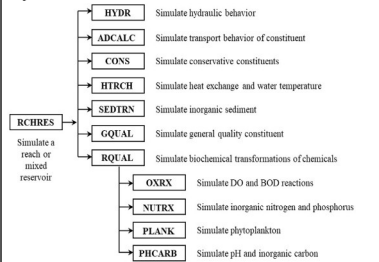
圖 5 RCHRES 模組之架構
