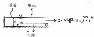
圖 1 非線性蓄水模型示意
