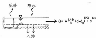
圖 1 非線性蓄水模型示意
