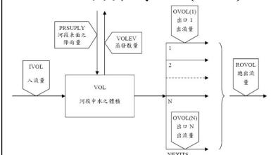
圖8 HYDR 副程式之演算流程
