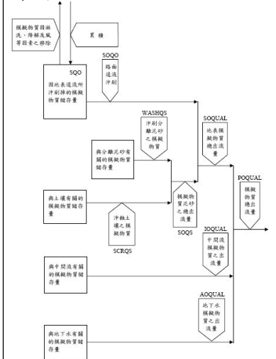
圖 11 PQUAL 副程式之演算流程
